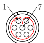
公针芯焊接端 焊接排序图
