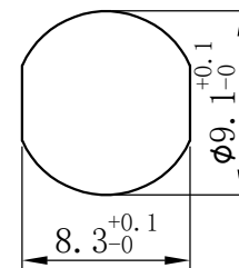
面板开口尺寸
