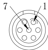
母针芯焊接端 焊接排序图
