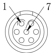
公针芯焊接端 焊接排序图
