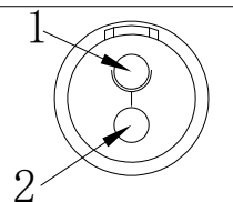
公针芯焊接端 焊接排序图
