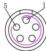
母针芯焊接端 焊接排序图
