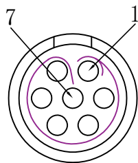
母针芯焊接端 焊接排序图
