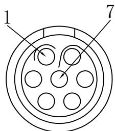
公针芯焊接端 焊接排序图
