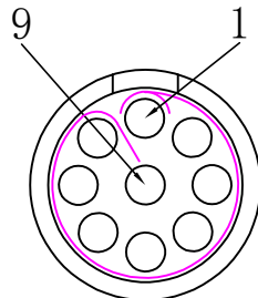
母针芯焊接端 焊接排序图
