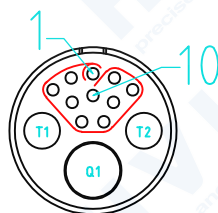
公针芯焊接端 焊接排序图
