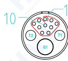
母针芯焊接端 焊接排序图
