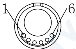
公针芯焊接端 焊接排序图
