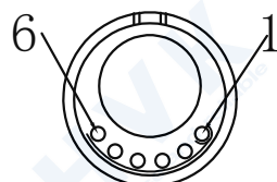
母针芯焊接端 焊接排序图
